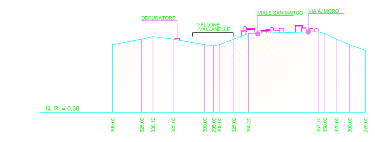
PROFILO E
