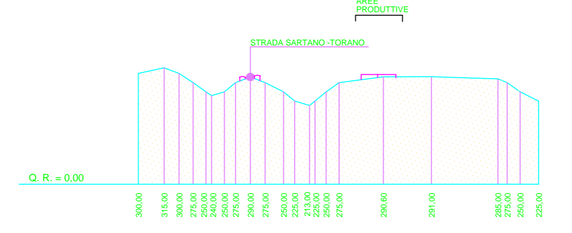
PROFILO G
